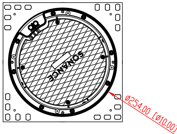
TRIMLESS GRILLE
